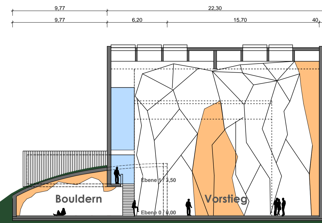
Querschnitt Bouldern 1/200
