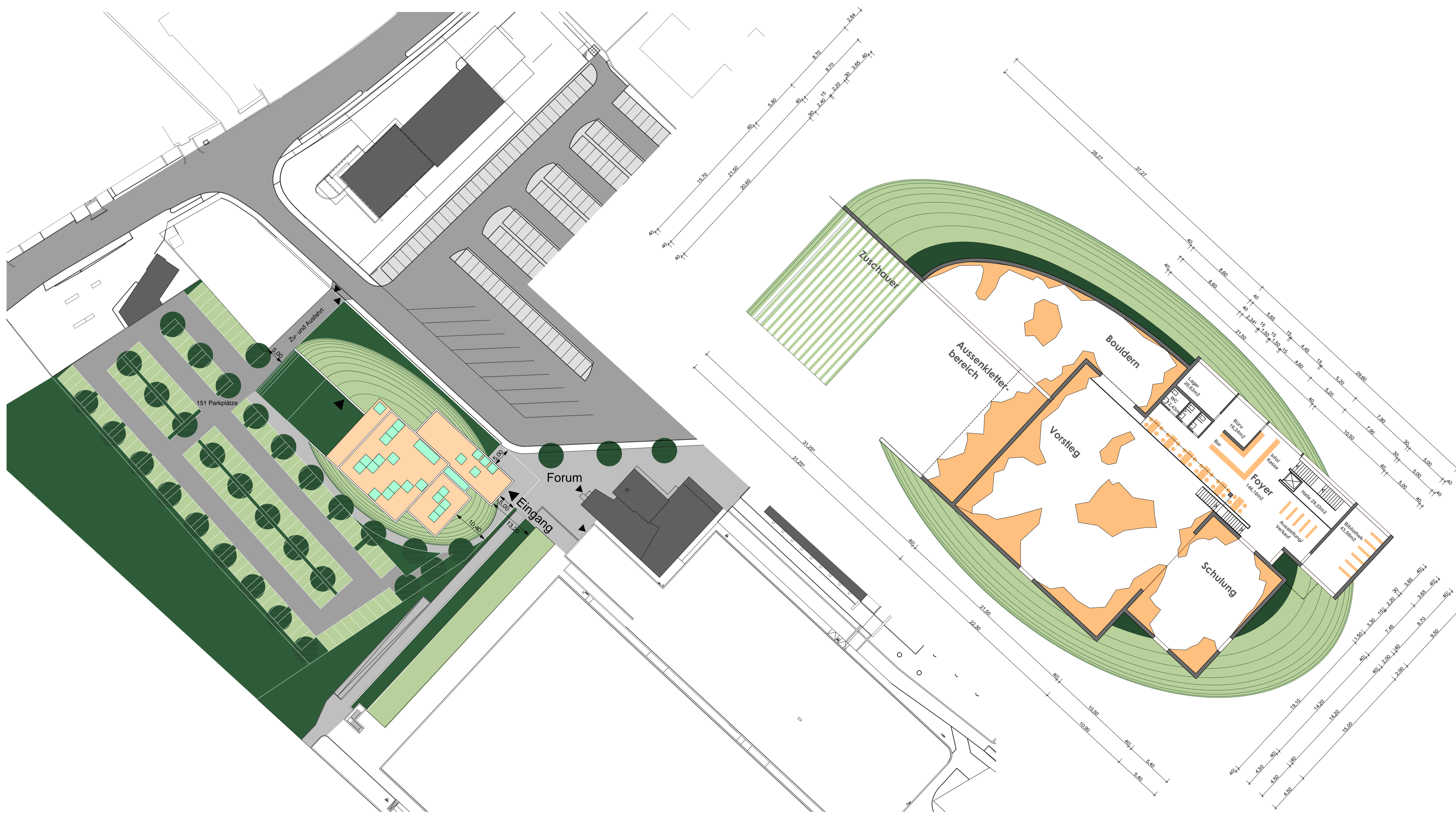
Lageplan 1/500
