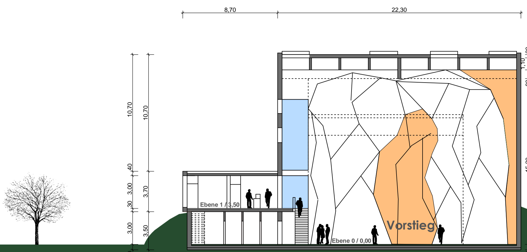
Querschnitt Eingang 1/200
